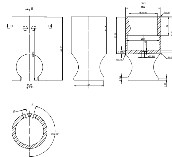
EMPORIA-040901 Uchwyt na słuchawkę
