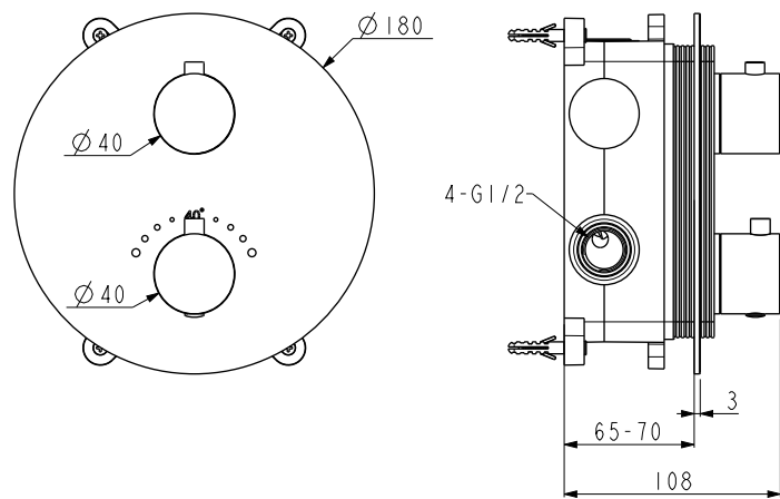
EMPORIA-03043 Bateria prysznicowo-wannowa
