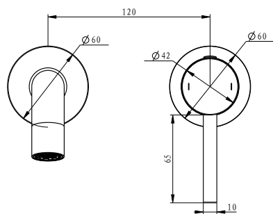
EMPORIA-03012 Bateria umywalkowa
