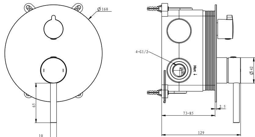
EMPORIA-03042 Bateria prysznicowo-wannowa
