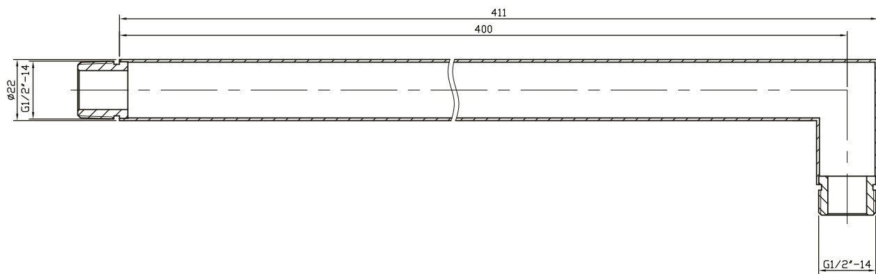
EMPORIA-04050 Ramię deszczownicy
